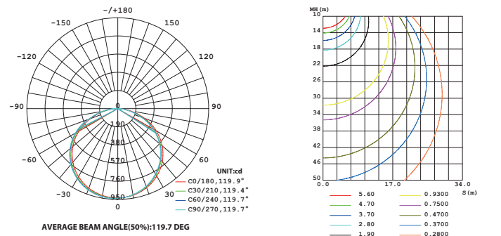
Diagramme de distribution de l'intensité lumineuse Diagramme (Unit : lx) C0 plan Isolux
